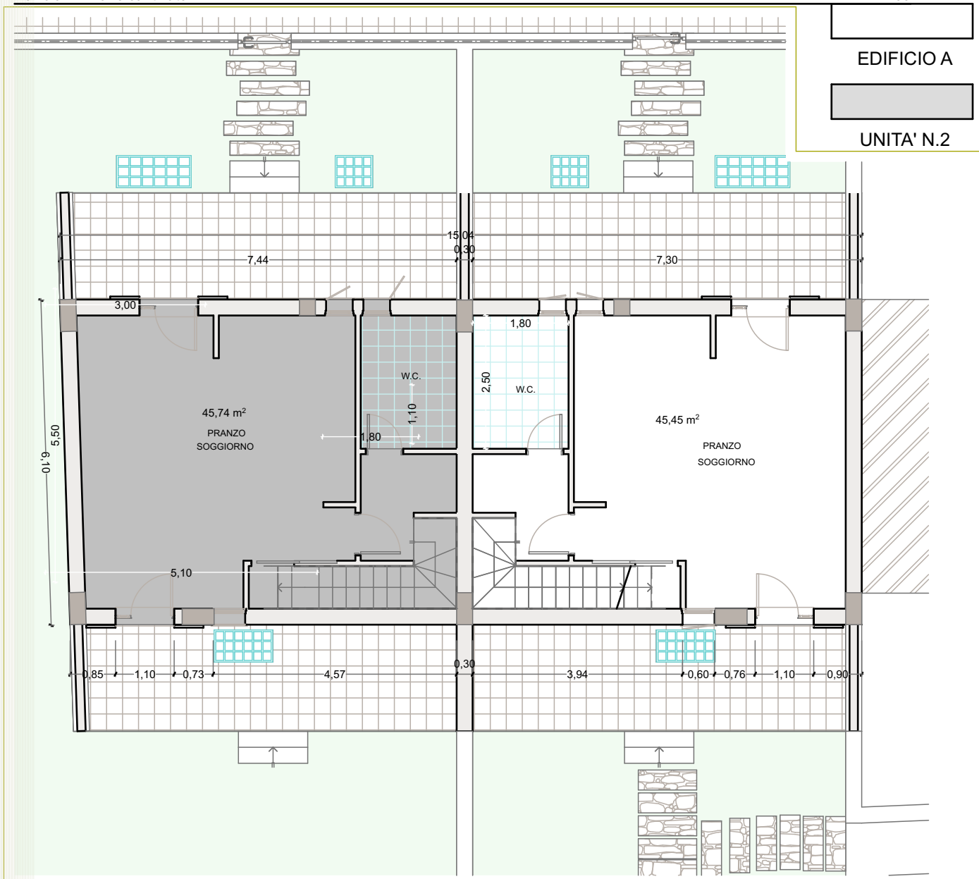
Edificio A - Piano terra
