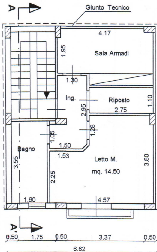
PIANTA SECONDO PIANO
