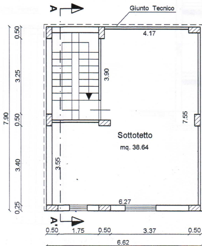
PIANTA TERZO PIANO SOTTOTETTO
